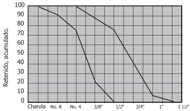
GRANULOMETRÍA GRAVA 5 A 25 mm
