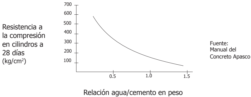
Figura 6 EFFECTO DE LA RELACIÓN AGUA/CEMENTO EN LA RESISTENCIA A LA COMPRESIÓN DEL CONCRETO
