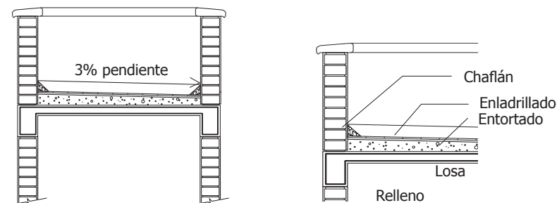
Figura 23 SISTEMA DE ESCURRIMIENTO EN LOSA-TAPA
